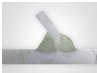
Macrografia de solda robotizada em junta complexa de componente automotivo. Aço-carbono 1020, em espessuras de 3mm e 6mm.
